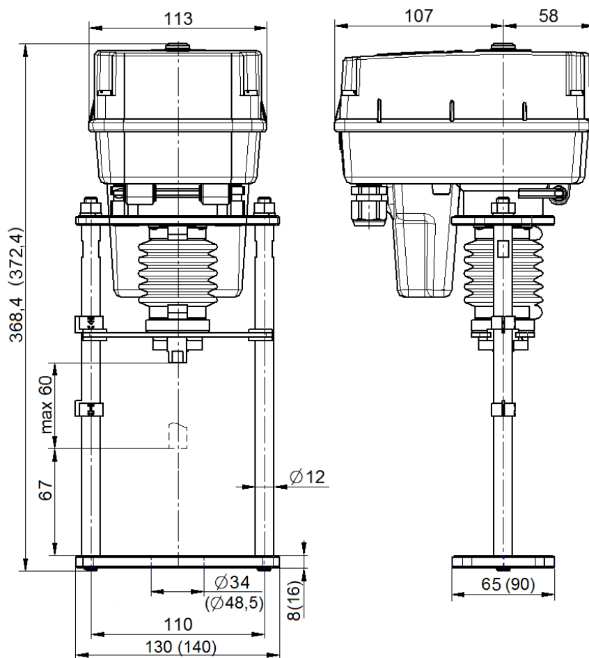
Рисунок А.4 Присоединительные размеры электропривода TSL-3000-1-230 и TSL-3000-1R-230 во фланцевом исполнении
